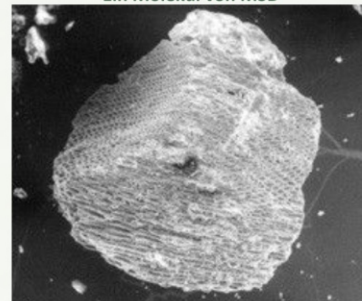
Ein Molekül von MSD
